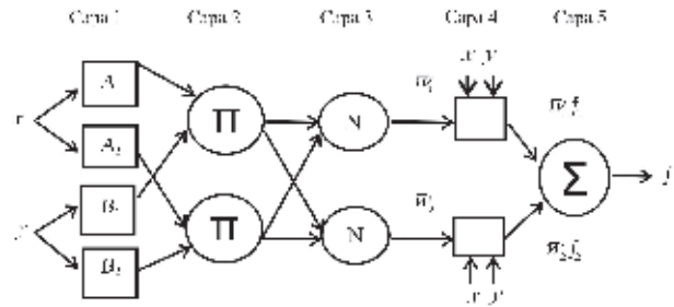
Figura 2 Red ANFIS
